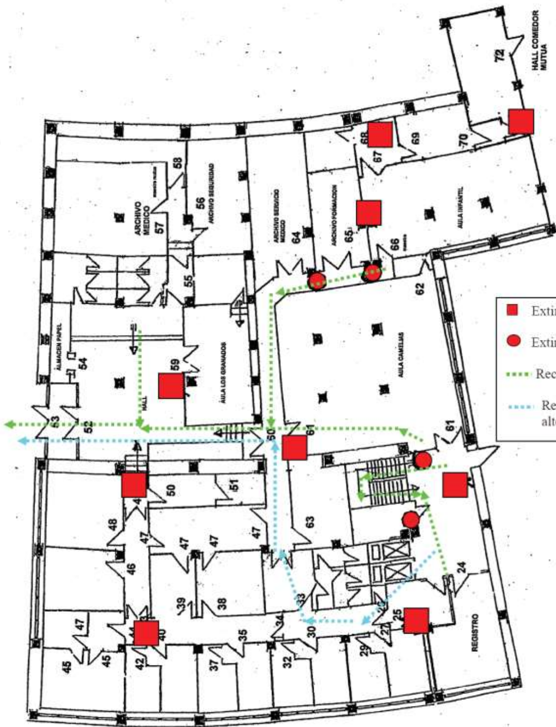
Planta -1
